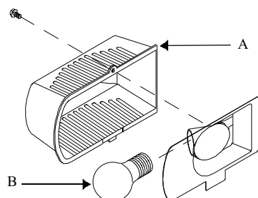
A. Cubierta del foco
